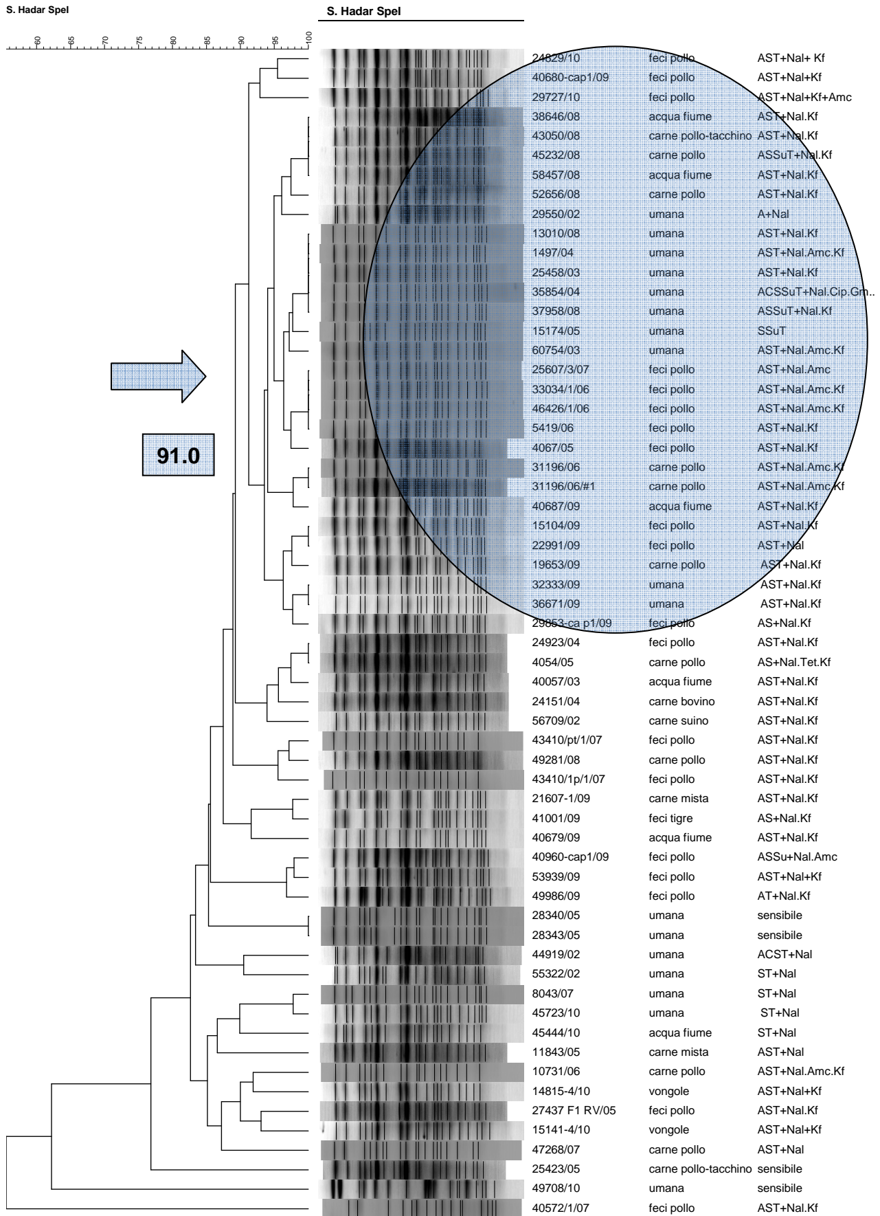
Figura 1. Cluster analysis dei 60 ceppi analizzati. In evidenza il cluster con omologia \geq 90\% ; digestione eseguita con l'enzima SmaI.
